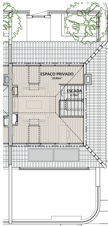
SOTÃO
