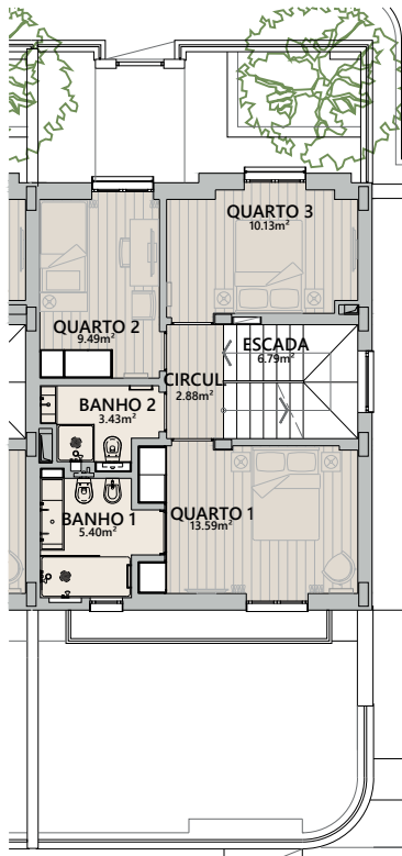
PISO 1
