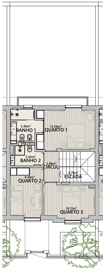
PISO 1
