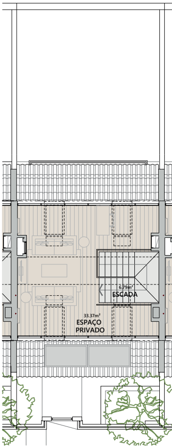
SOTÃO
